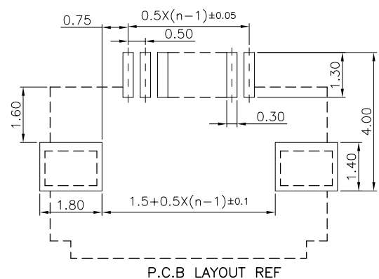
P.C.B LAYOUT REF
