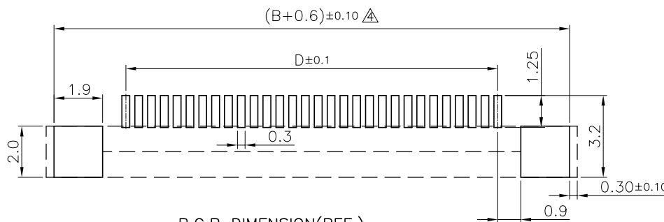
P.C.B DIMENSION(REF.)
