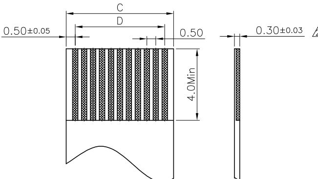
F.P.C DIMENSION(REF.)
